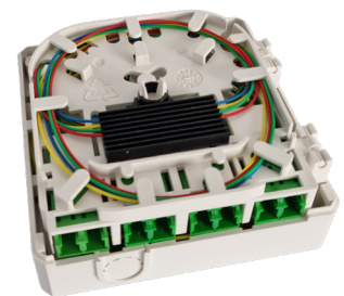
CCM ARCA FTTH XS Anschlussdose bestückt mit 4 LCAPC Duplex Kupplungen
