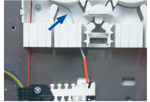
6H Kabel 10 mm unterhalb des Bündeladerhalters absetzen. Bündelader 10 mm oberhalb des Bündeladerhalters abisolieren und einführen.
