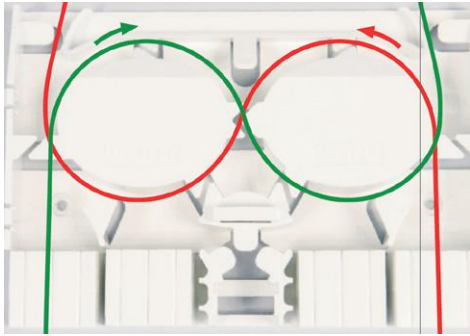
6J Beispielhafte Faserführung im Mixer. Absetzlänge der Fasern ca. 2 m.
