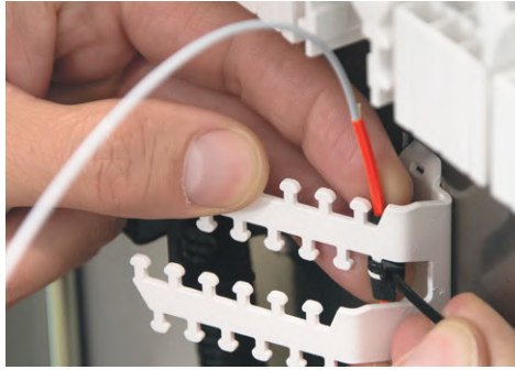
6G Kabel bis zur Bündelader abisolieren und mit Kabelbinder an Abfangung befestigen. Tipp: Beginnen Sie mit dem hintersten, innersten "T-Zapfen". Material: Kabelbinder 96/2,5 mm (Art. Nr. 970333)
