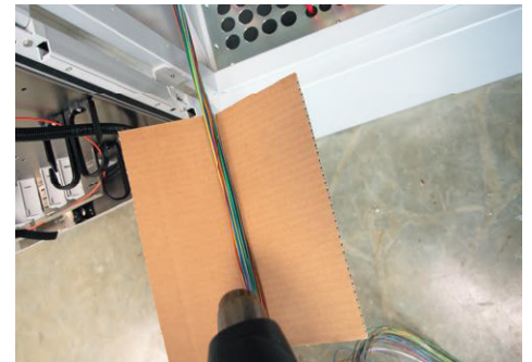
4F Bündelader mit Heissluft glätten und in den Wellschlauch einführen. Tipp: Zur Erzielung eines besseren Glättungsergebnisses, einen geknickten Karton unter den Bündeladern platzieren. Achtung! Bündeladern nicht zu heiss föhnen, um Beschädigungen zu vermeiden.
