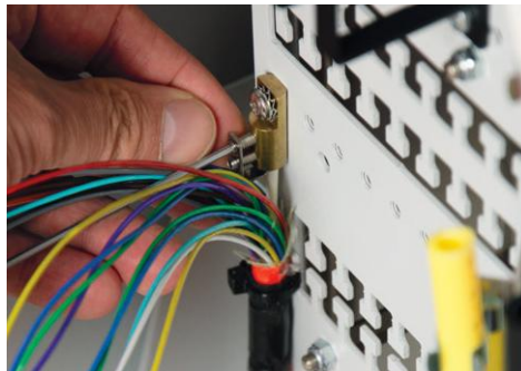
4E Abfangung auf Zentralelement stecken und anschliessend Abfangung auf Kabelabfangplatte befestigen. Madenschrauben an Abfangung anziehen. Tipp: Abfangung ausserhalb der Kabelachse setzen, so dass die Bündeladern an der Abfangung vorbeilaufen. Werkzeug: PH1 Schraubendreher, Innensechskantschlüssel 2 mm
