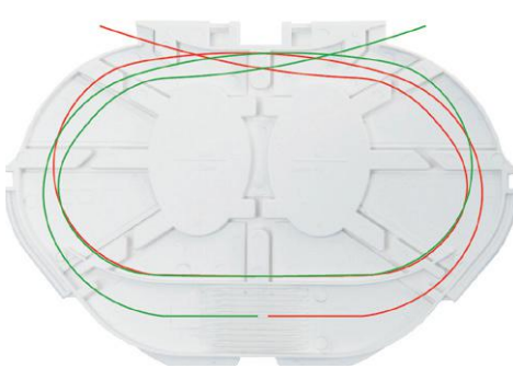
6K Faserführung in der Spleisskassette.
