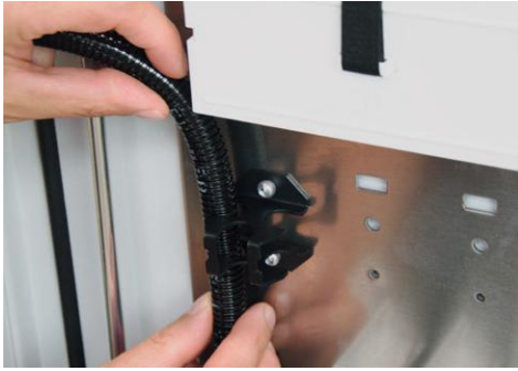
3E Flexschlauch unterhalb des Mixers in Halterung positionieren.
