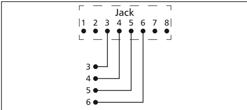
Schaltbild 906806 Connection Diagram 906806
